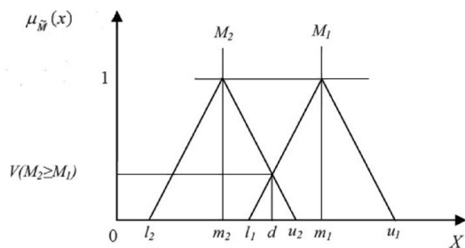
شكل شماره ٤: محاسبه درجه بزرگى دو عدد فazy نسبت به يكدیگر
