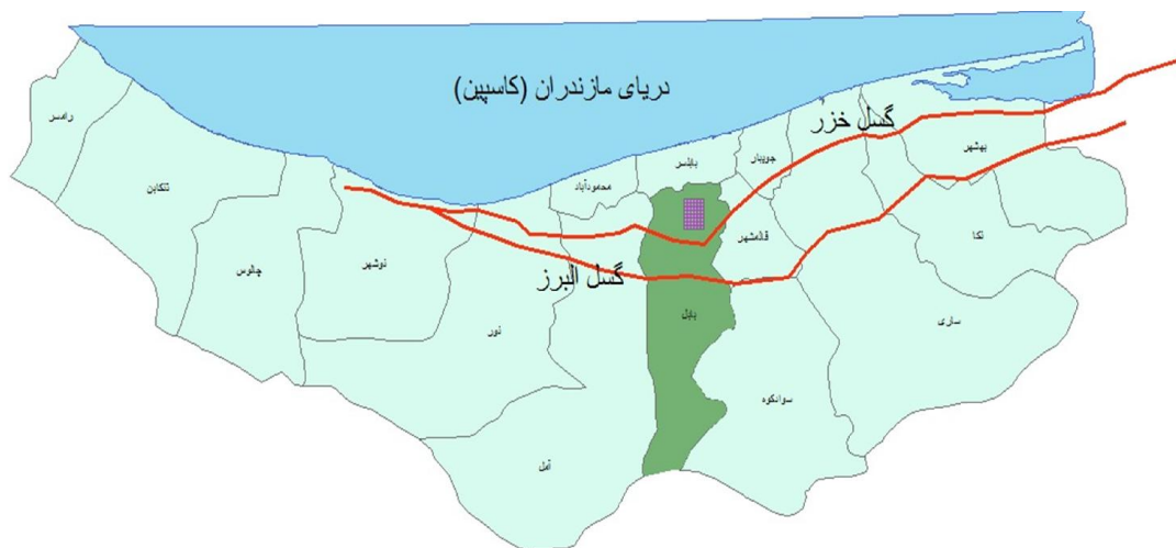
شکل شماره ۱: محدوده مورد مطالعه و گسل‌های آن
