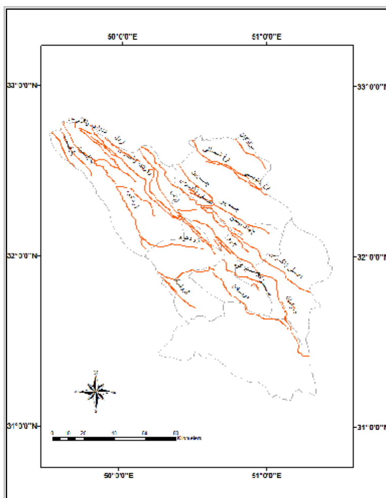
شکل شماره ۲- وضعیت گسل‌های فعال در استان چهارمحال و بختیاری
